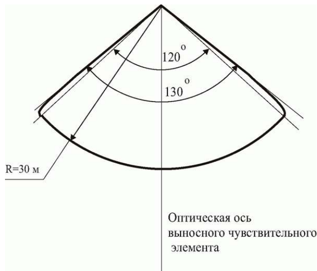
Рис. 1. Проекция поля зрения выносного чувствительного элемента извещателя "Пульсар 3-013"
