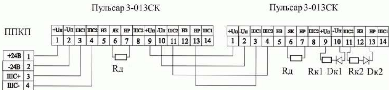
Рис. 8а Монтажная схема последовательного подключения “Пульсар3-013НК”, “Пульсар3-013СК” С нормально разомкнутым контактом реле
