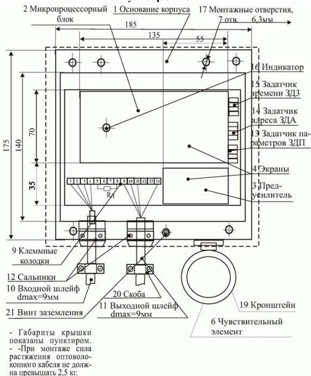
Рис. 2. Извещатель пожарный пламени "Пульсар 3-013" вид со снятыми крышкой и защитной пластиной
