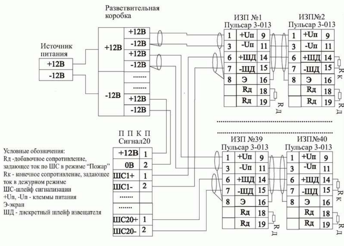
Рис. 5. Схема подключения извещателей "Пульсар 3-013Н" "Пульсар 3-013С" на примере ППКП "Сигнал 20"
