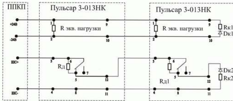
Рис. 7б Принципиальная схема последовательного подключения “Пульсар3-013НК”, “Пульсар3-013СК” с нормально замкнутым контактом реле.
