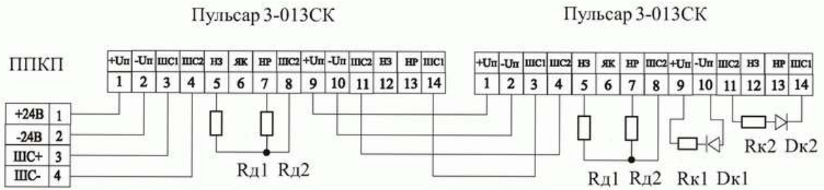
Рис. 6а Монтажная схема параллельного подключения “Пульсар3-013НК”, “Пульсар3-013СК”.
