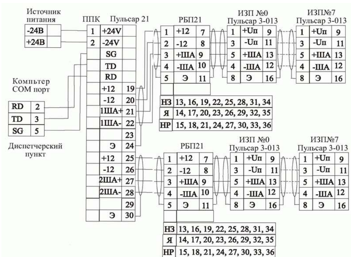
Рис. 4. Схема подключения извещателей "Пульсар 3-013Н", "Пульсар 3-013С" к ППКП "Пульсар 21"
