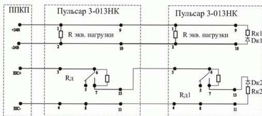
Рис. 8б Принципиальная схема последовательного подключения “Пульсар3-013НК”, “Пульсар3-013СК” С нормально разомкнутым контактом реле
