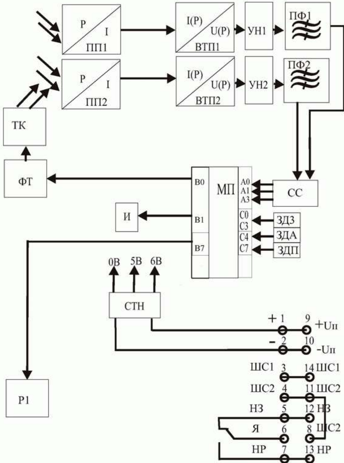
Рис. 3. Схема функциональная извещателя "Пульсар 3-013СК"
