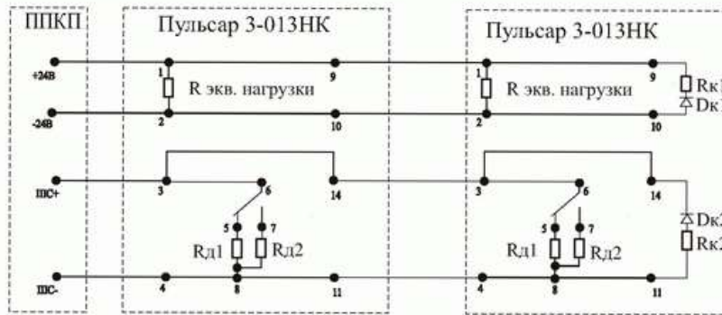
Рис. 6б Принципиальная схема параллельного подключения “Пульсар3-013НК”, “Пульсар3-013СК”.
