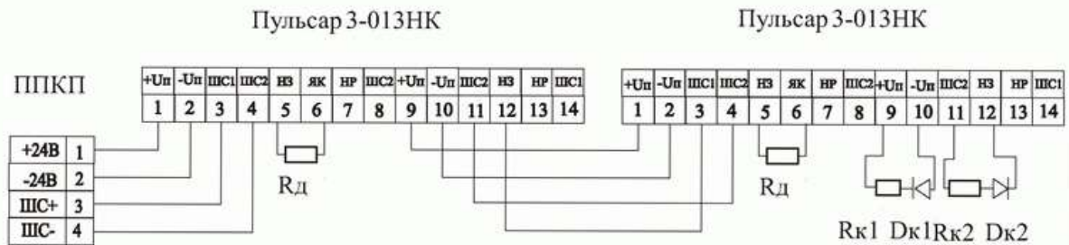
Рис. 7а Монтажная схема последовательного подключения “Пульсар3-013НК”, “Пульсар3-013СК” с нормально замкнутым контактом реле.
