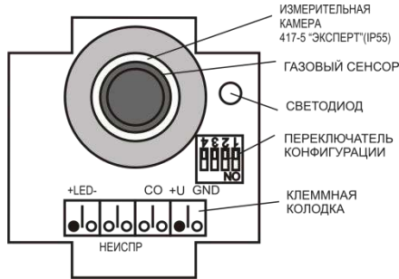
Рис.1 - Расположение основных элементов на плате ИП417-5 «Эксперт» (IP55)
