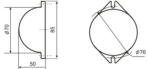
Рис.1. Габаритные и установочные размеры
