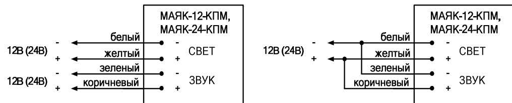
Рис.1. Схема подключения.
