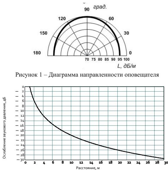
Рисунок 2 – Зависимость ослабления уровня звукового давления от расстояния до оповещателя
