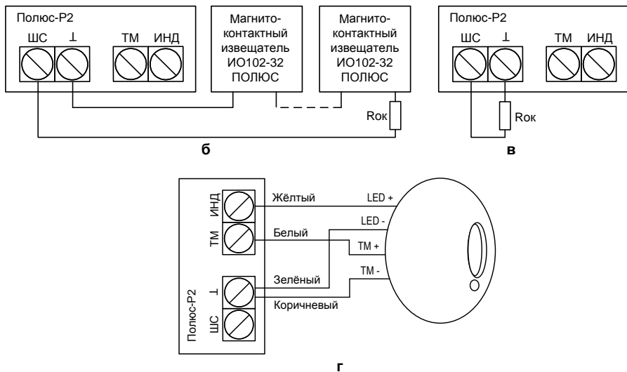
Рис.11б, в, г Схемы подключений к Полус-Р2
