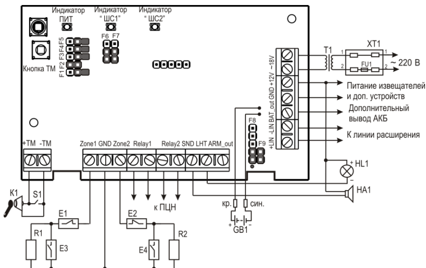
Рисунок А.1- Схема подключения «РПУ Астра-Р» исполнение Б
