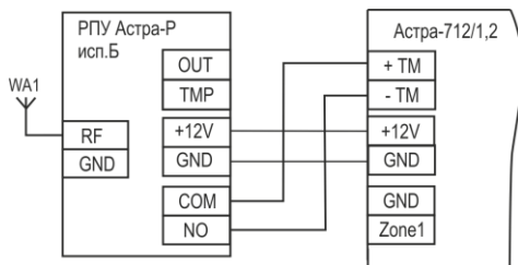
Рисунок А.1- Схема подключения «РПУ Астра-Р» исполнение Б
