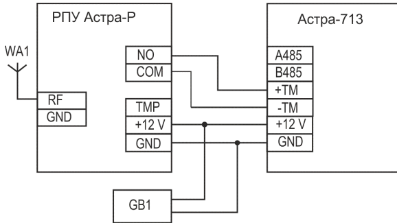
Рисунок А.1 - Схема подключения «РПУ Астра-Р»
