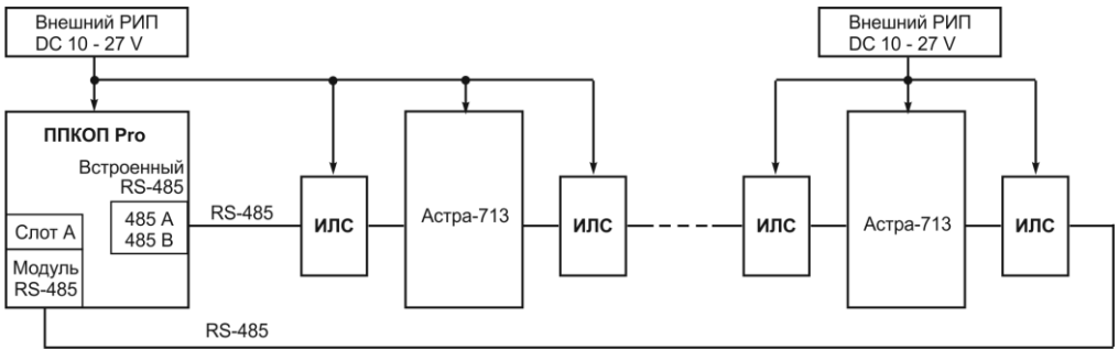
Рисунок Б.2 - Общая схема подключения прибора «Астра-713» в «кольцо» по интерфейсу RS-485 с использованием изоляторов «Астра-А ИЛС»
