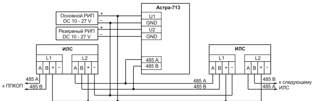
Рисунок Б.3 – Схема подключения изоляторов «Астра-А ИЛС» к прибору «Астра-713»
