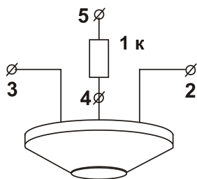
Рис. 5. Организация двухпорогового шлейфа пожарной сигнализации
