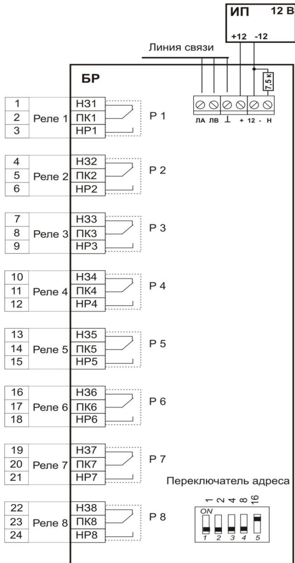
Рис 2. Схема внешних соединений блока реле
