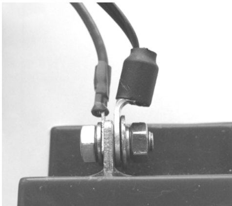
Подключение термодатчика.
