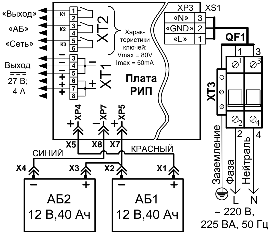
Схема подключения РИП
