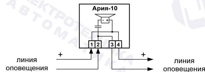
Рис.1. Схема подключения.
