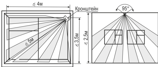
В) Вариант установки в оконном проеме
