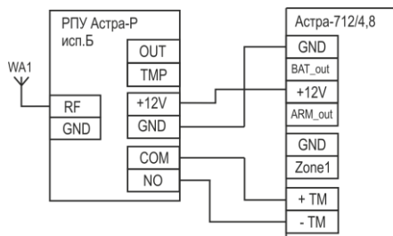
Рисунок А.3 - Схема подключения «РПУ Астра-Р» исполнение Б
