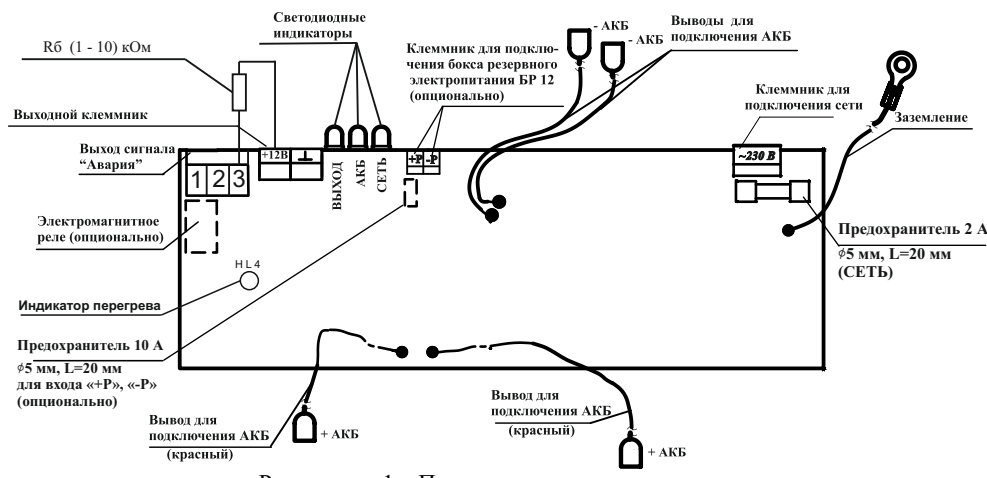
Рисунок 1— Плата источника
