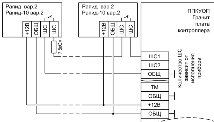
Рис.Б4 Схема подключения охранных извещателей Rapid вар.2, Rapid-10 вар.2
