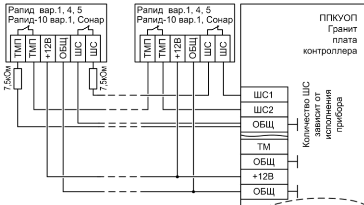
Рис.Б3 Схема подключения охранных извещателей Rapid вар.1,4,5, Rapid-10 вар.1, Сонар (тампер подключён к отдельному ШС)
