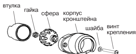
Рисунок 2 – Детали кронштейна
